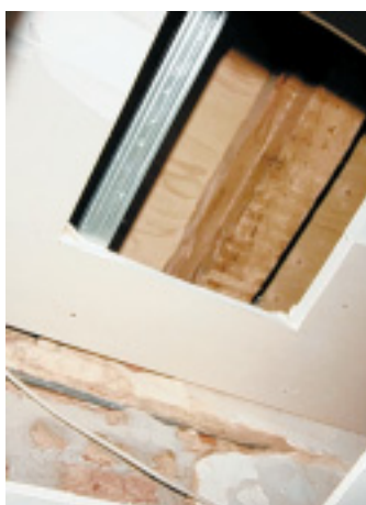
Fehlerhaft: Die Decke zwischen Erd- und Obergeschoss. Sie würde einem Feuer nicht standhalten.
